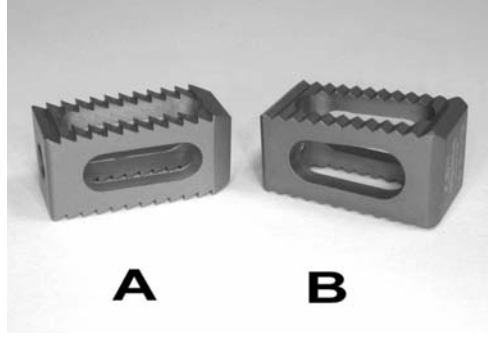
Şekil-6. Dikdörtgen kafeslerin tüm yüzeylerinde geniş oluklar bulunur. Verilmek istenen lordoz miktarına göre tam dikdörtgen (A) veya öne doğru genişleyen tasarımlarda (B) seçenekler bulunur.
